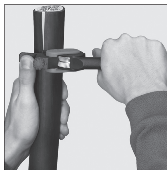
Drehen des Werkzeugs für Umfangsschnitt Turning the tool for circumferential cut
