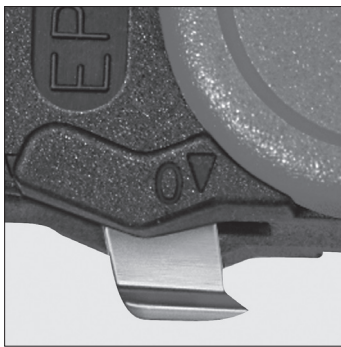
Einstellbare Schnitttiefe Adjustable cutting depth
