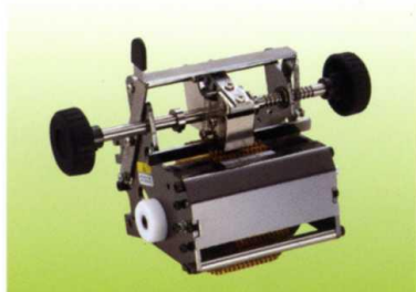
Tisková hlava G (systém volících koleček)
