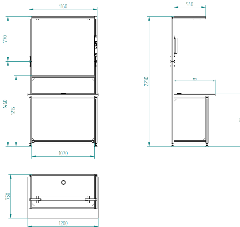
Abbildung: Abmessungen Handarbeitsplatz HA-1200 (ohne Auf- und Anbauten)
